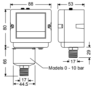
Méreték
